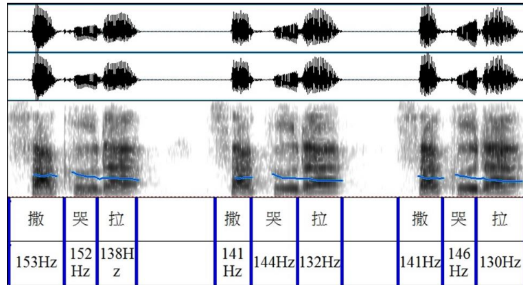
(圖 4)「撒哭拉」的頻率
