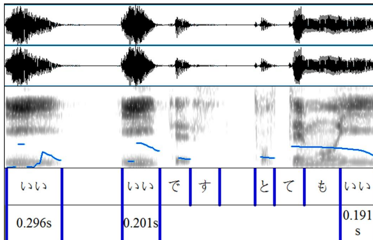
(圖一)「いい」的時間值
