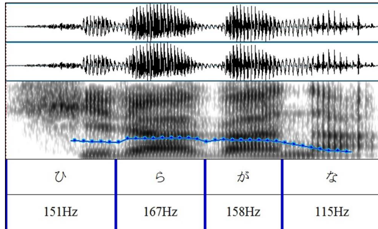
(圖5) 「ひらがな」高低音調變化
