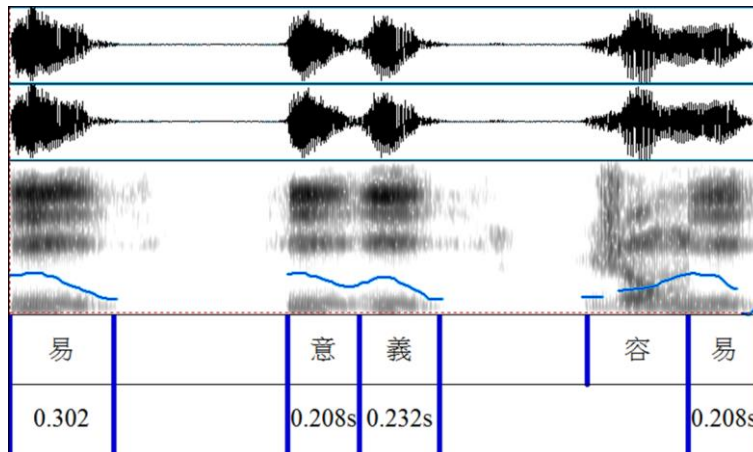
(圖二)「易・意・義」的時間值
