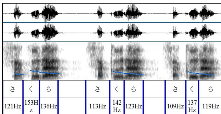
(圖3)「さくら」的頻率
